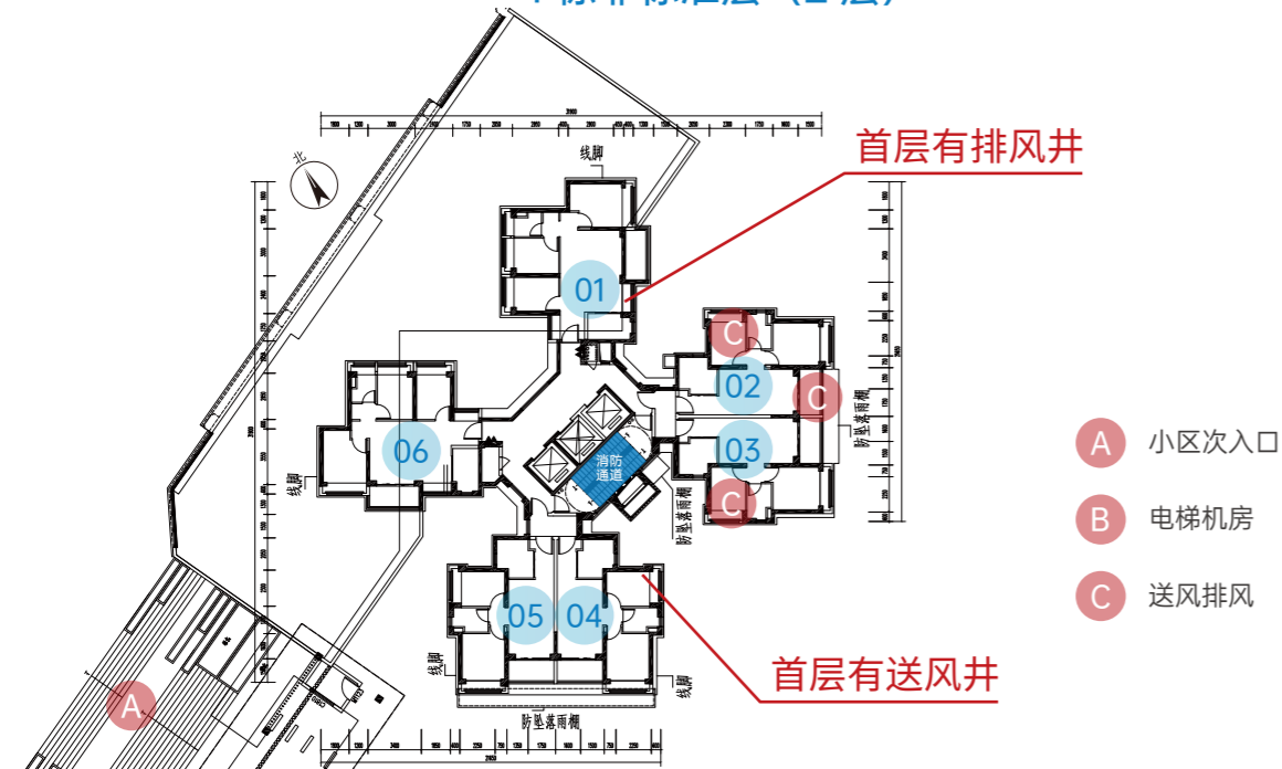
4栋非标准层 (2层)
