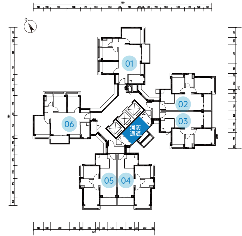
4~5栋标准层 (3-16、18-33、35-51层)
